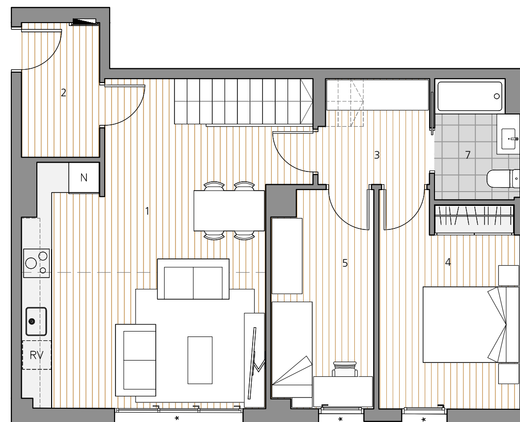
PLANTA BAIXA
